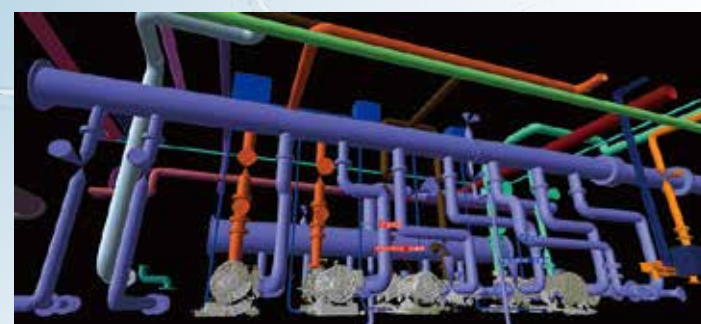
3D-CADモデル
